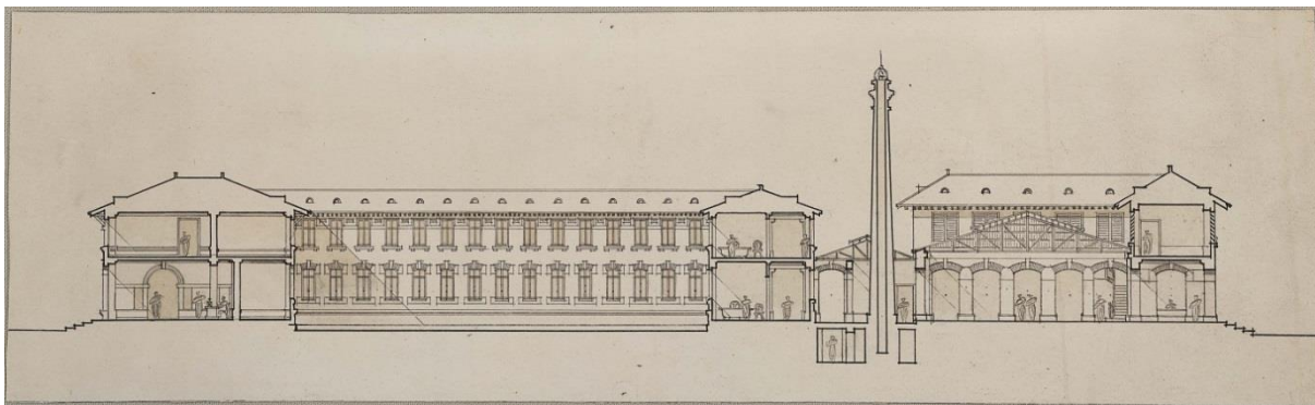
162 J 75 plan 1, coupes du bâtiment des abattoirs de Lons (projet).
